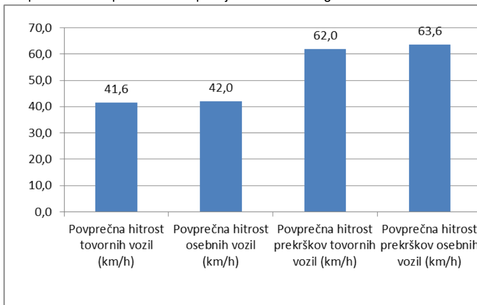
Graf 4: Prikaz povprečne hitrosti po posamezni vrsti vozil
